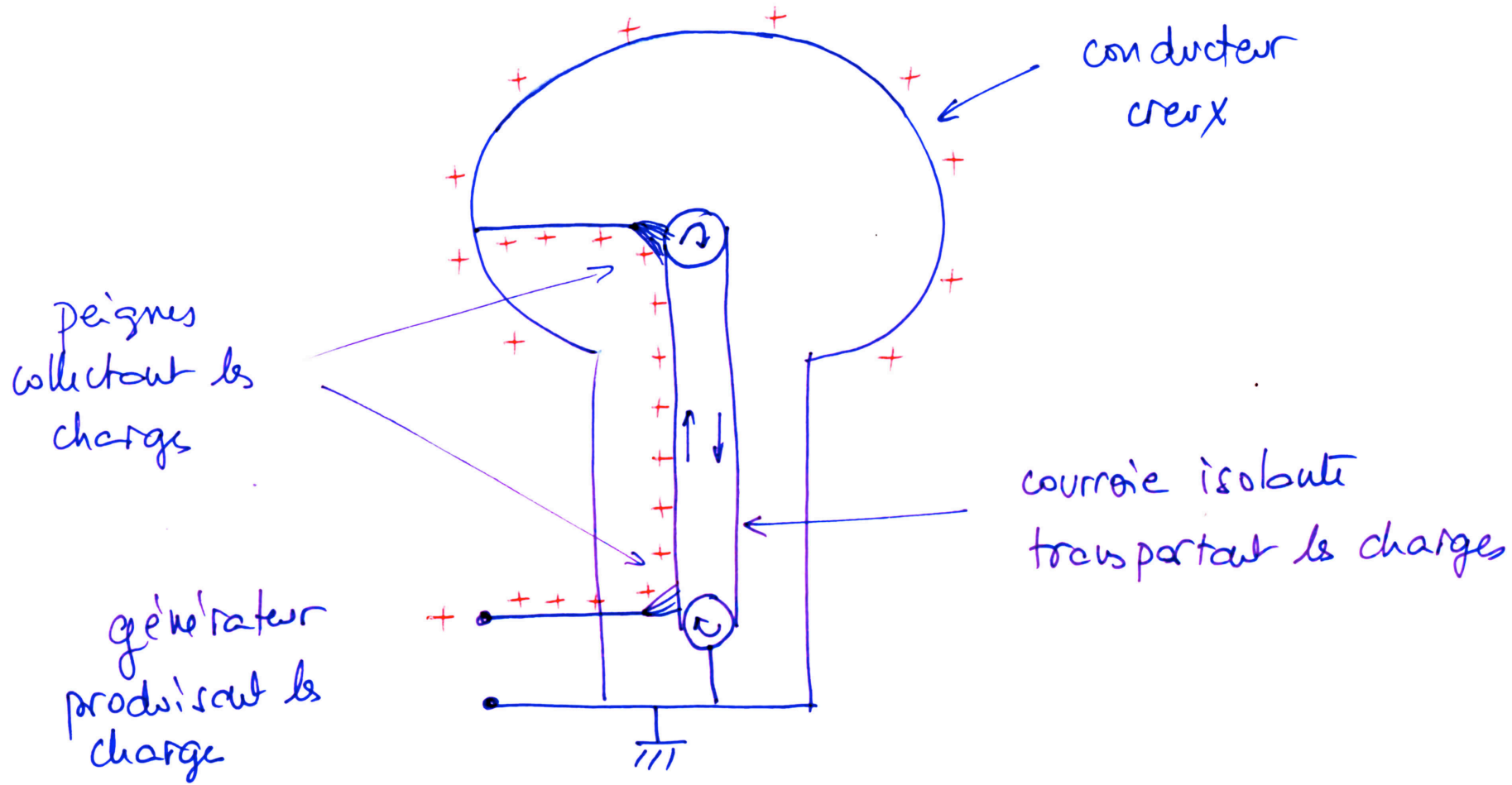
Le générateur de Van de Graaff
