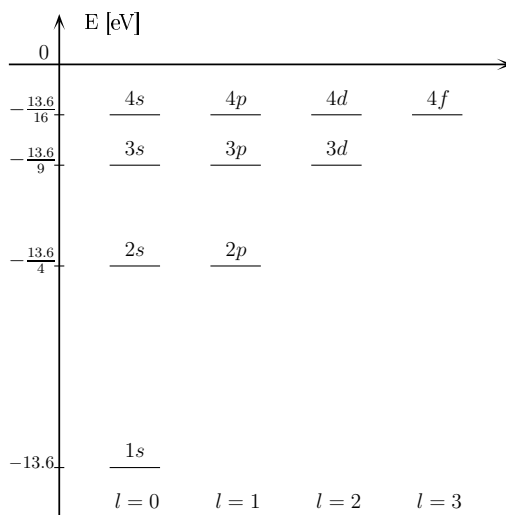
FIG. 2 – Les 6 premières fonctions d'ondes de l'oscillateur harmonique 1d
