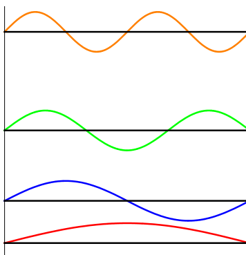
FIG. 1 – Les 4 premières fonctions d'ondes d'une particule dans un puits infini 1d
